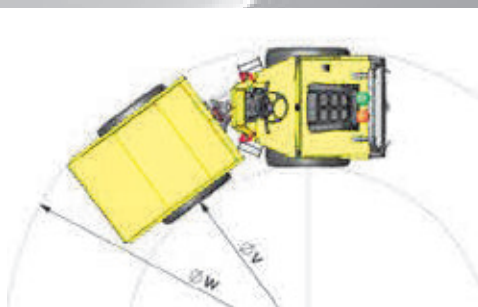
Statische Abmessungen (mm)
